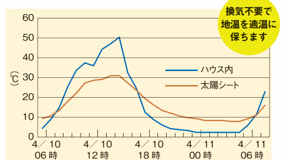
「本州太陽シート」の温度データ 新潟県長岡市(2017年) 本データは実測値であり保証値ではありません
